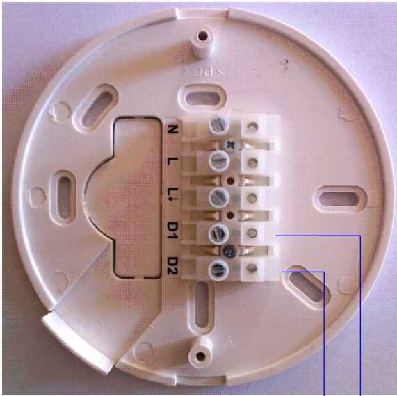
PIR-sensor
