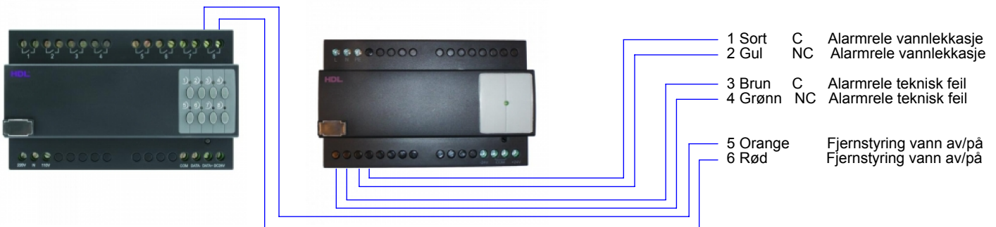
Kabel fra dørbryter
